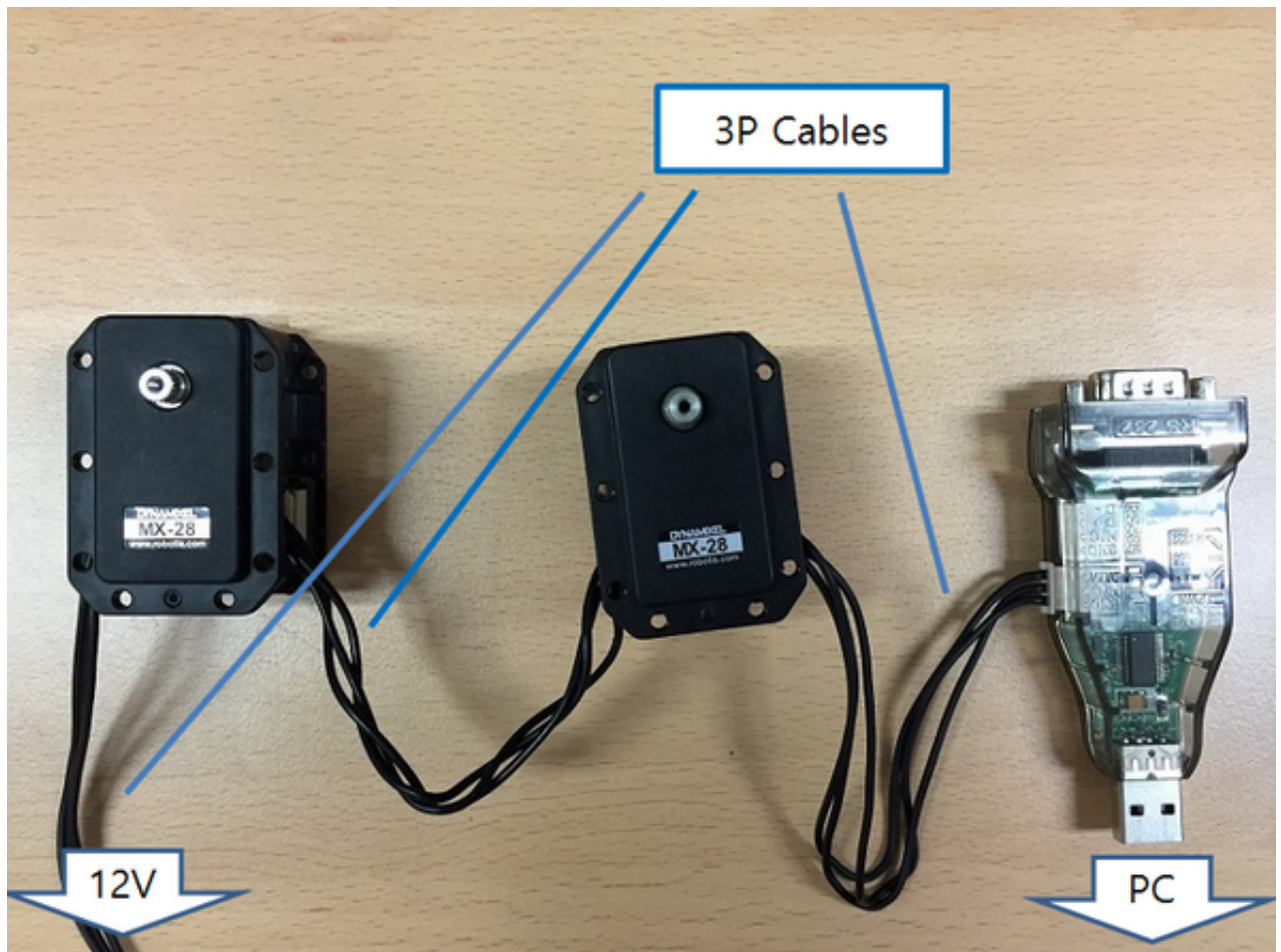
Figura 4.4: Conexão para os dynamixels
