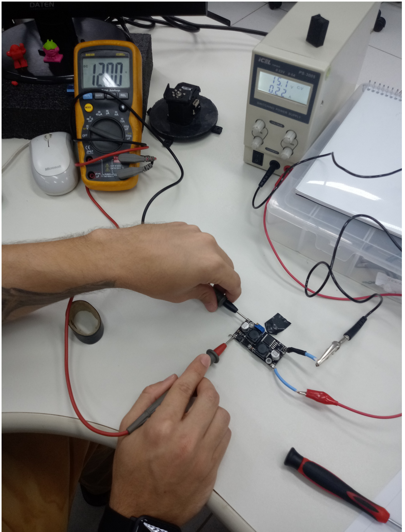
Figura 4.10: Calibração do conversor XL6019
