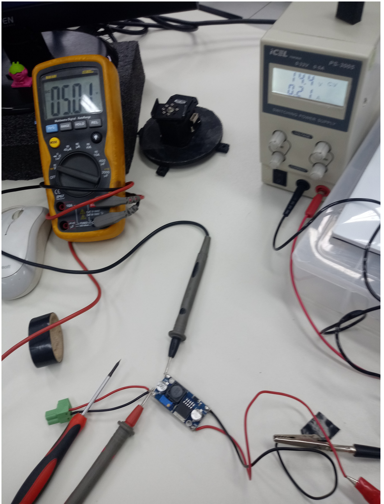
Figura 4.11: Calibração do conversor LM2596
