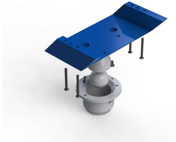
Figura 4.17: Peças da Roda Boba Fonte: Autores, 2019
