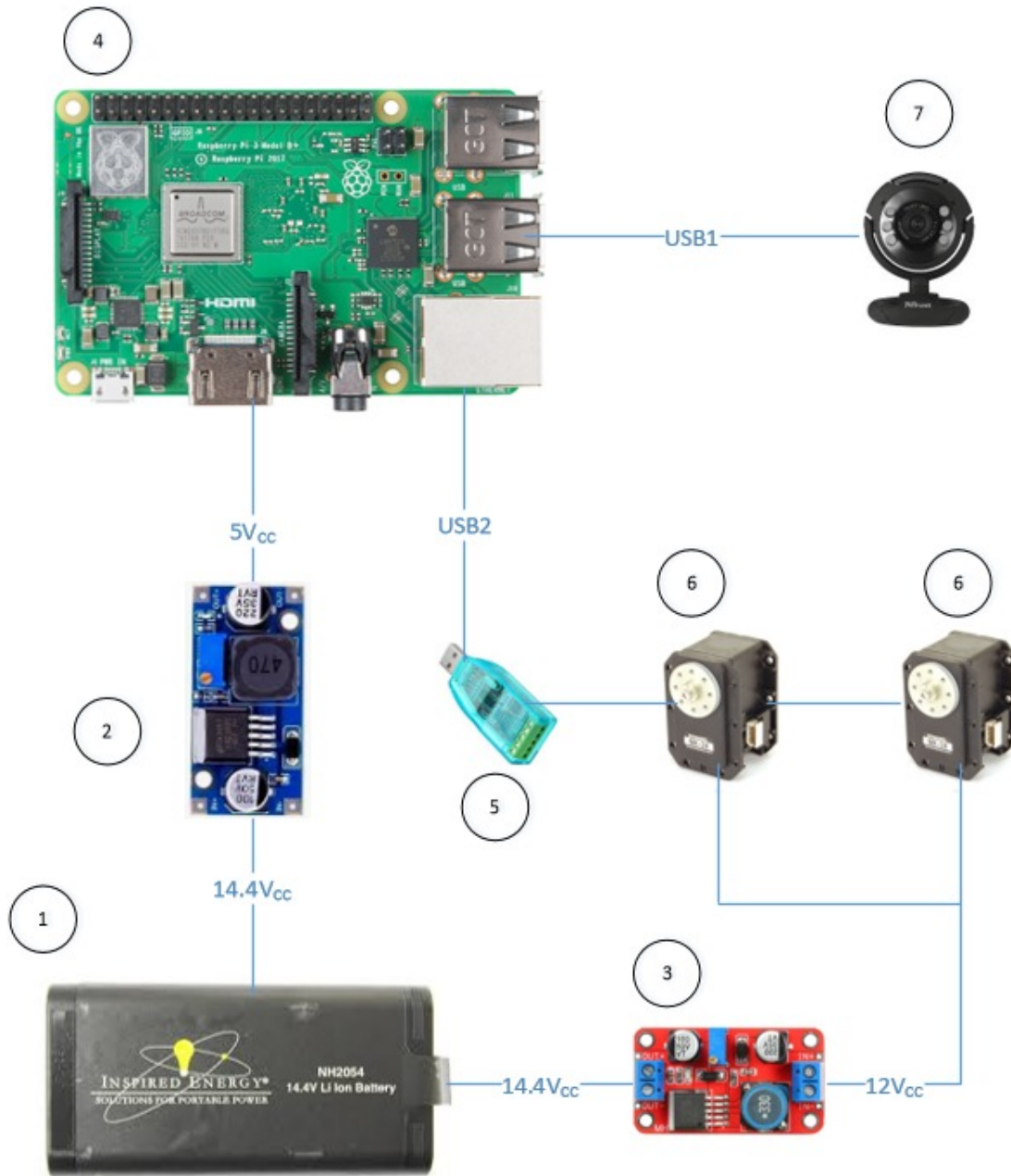
Figura 4.6: Esquema elétrico
