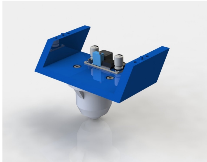
Figura 4.18: Montagem da Roda Boba Fonte: Autores, 2019
