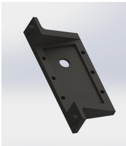
Figura 4.15: Peça Suporte Dynamixel Fonte: Autores, 2019
