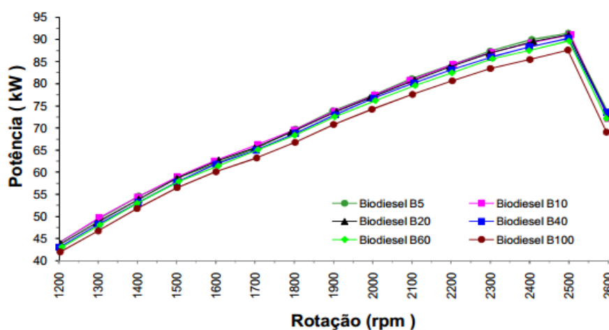
Figura 2. Potência versus Rotação das misturas de DM com biodiesel em proporções variadas 13
