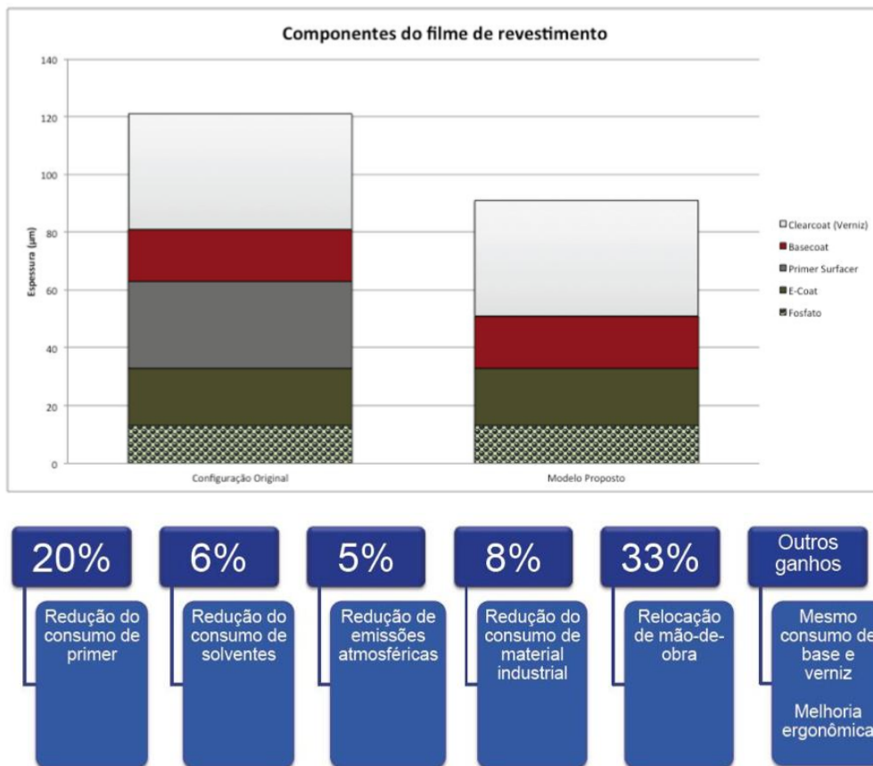
Figura 6. Camadas de pintura utilizadas num processo automotivo normal (esquerda) e com a proposta de eliminação da camada primer (direita) indicando os impactos avaliados na linha de produção 30
