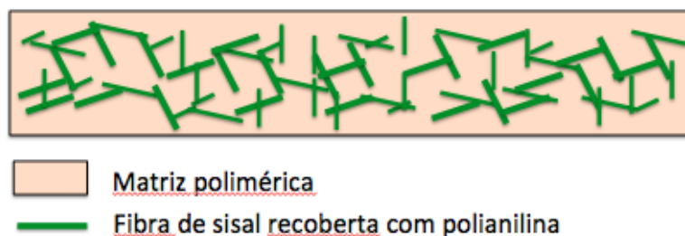
Figura 5. Mecanismo de condutividade elétrica em compósitos de matriz polimérica e fibras naturais modificadas com polímero condutor (polianilina) 8
